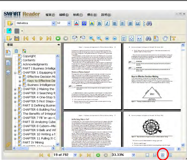
四頁瀏覽
