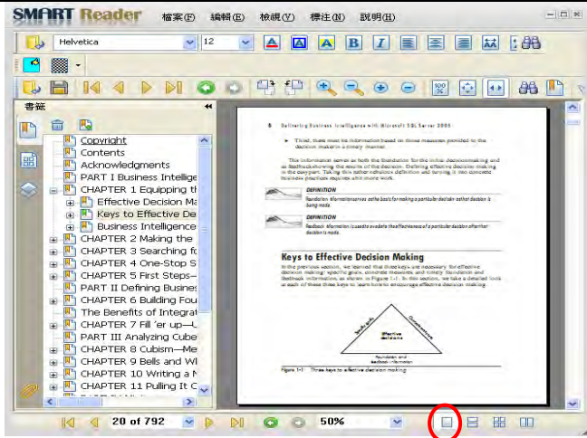
單獨頁面
