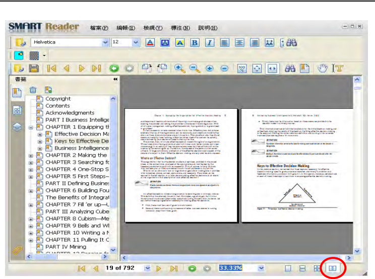
兩頁並排
